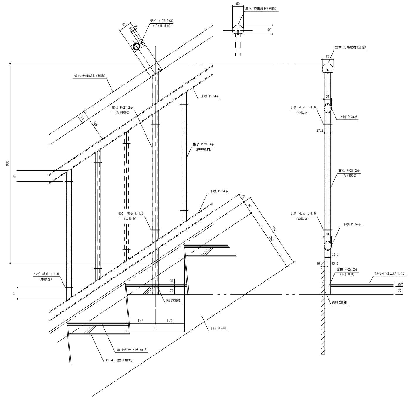
手摺詳細図 (階段) S=1/5
